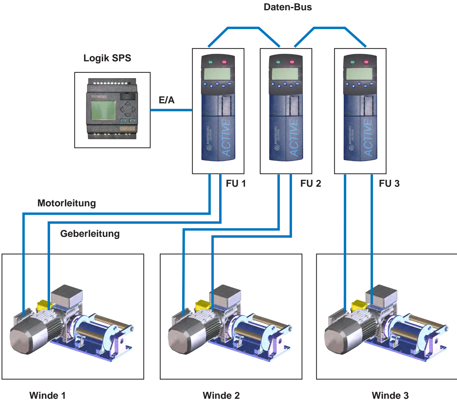
Prinzipverschaltung der Seilwinden „Elektronische Welle“
